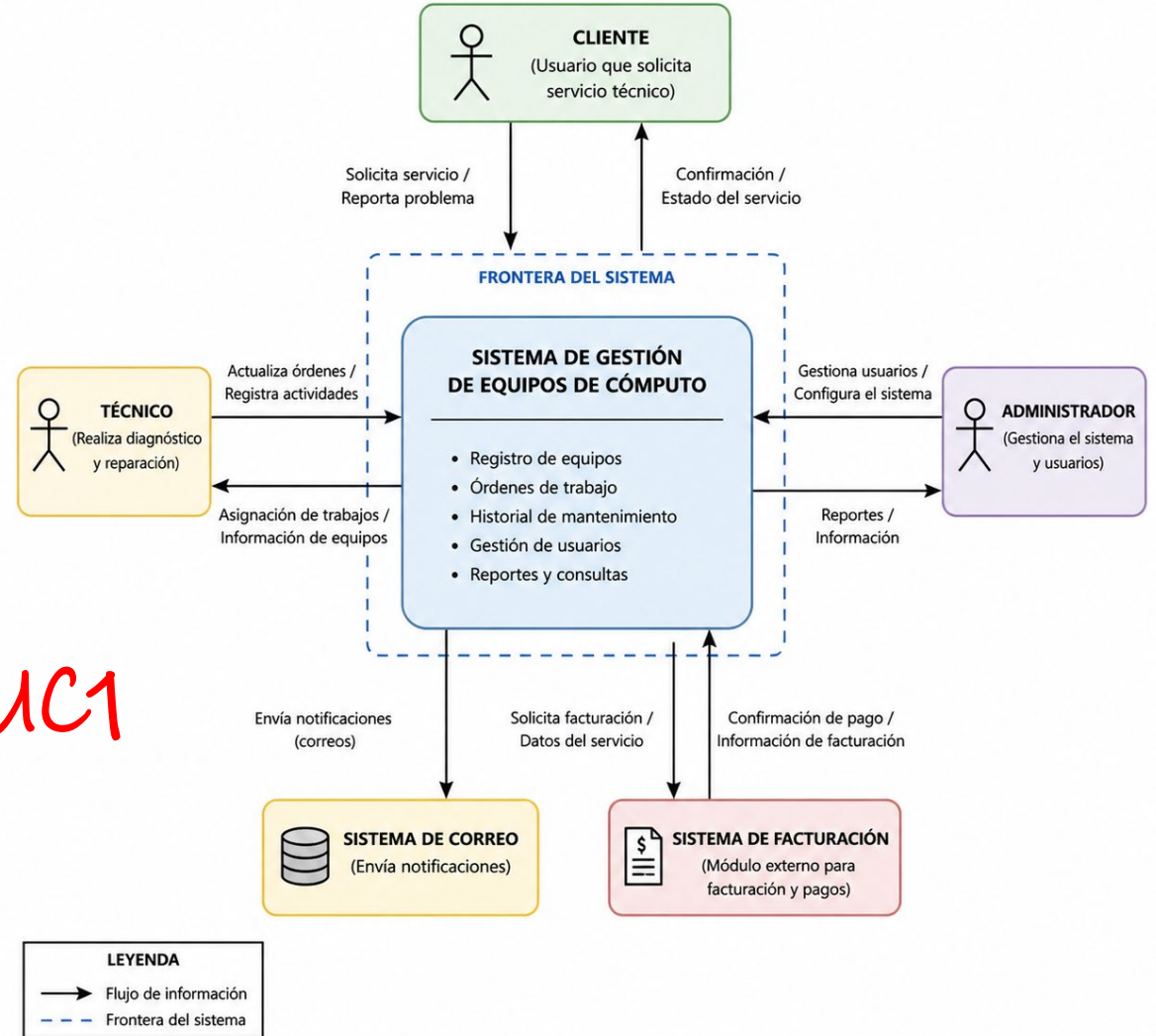
DIAGRAMA DE CONTEXTO (UML) Sistema de Gestión de Equipos de Cómputo
